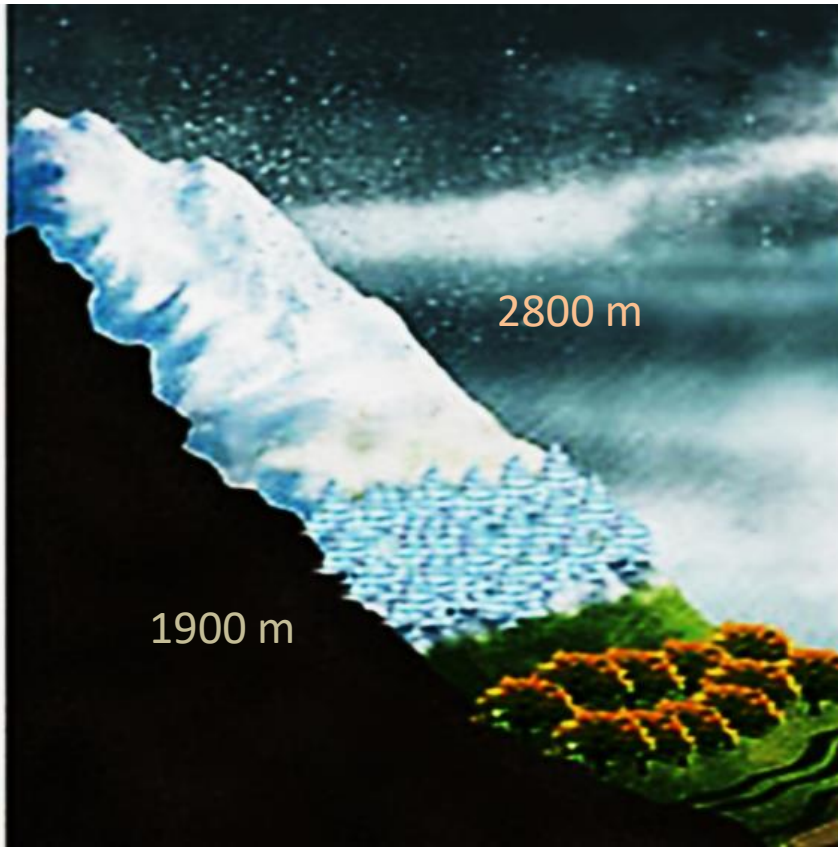
BAJO LA ACCIÓN DE UNA GLACIACIÓN
