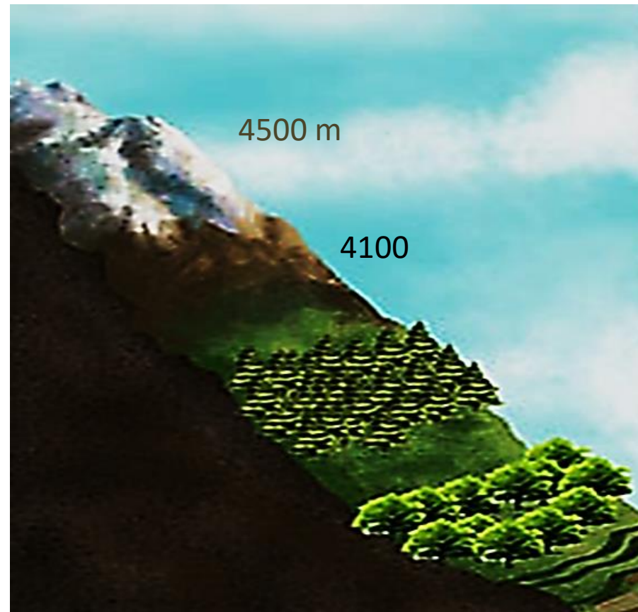
BAJO UNA INTERGLACIACIÓN
